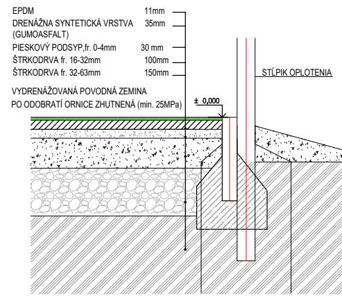
CHARAKTERISTICKÝ REZ M 1:100
